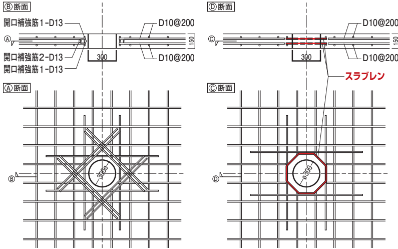
試験体の開口補強要領 (φ300の例)
